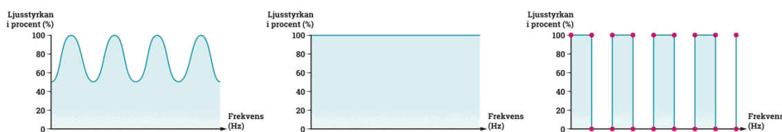
Figur 7.6 Olika ljuskällors ljusintensitetskurvor: sinuskurva och fyrkantsskurva. Fyrkantsskurvan ger upphov till ett svart randmönster över bilden när man tar foto med mobiltelefon (Illustration från Mynak (2021) Foto: Hillevi Hemphälä)
