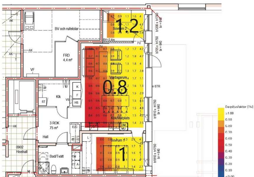
Figur 5.1 Dagsljusfaktorn har beräknats i ett rutnät av punkter och medianvärdet för varje beräkningsyta visas med större siffror. Värdena har överlagrats på planritning. Val av färgskala har gjorts så att alla punkter som överstiger myndighetskravet 1,0 % färgats gult. Detta underlättar tolkningen och kastar fokus på problemområden, som får successivt mörkare färg ju lägre resultat. (Källa: Fojab).
