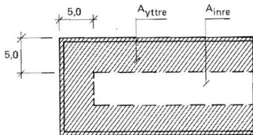
Figur 3.6 Reglering av högsta tillåten fönsterarea infördes i de nya energihushållningsreglerna i SBN 75, suppl. 1.
