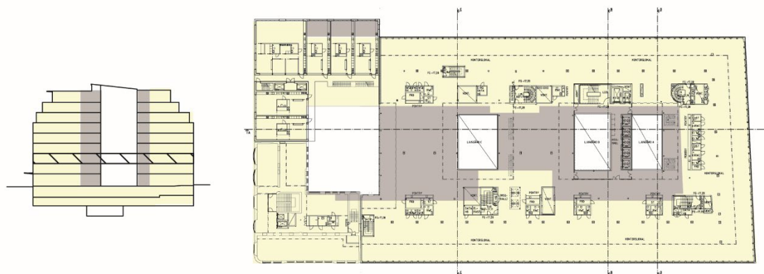
Figur 8.8 Renovering med ökade kontorsutrymmen (grått i figuren) på bekostnad av gårdsyta. Gula områdena i figuren visar ungefärlig byggnadsform på originalritningen från 1944. (sektion och planritningar Kv Träsket, Stockholm). (Källa: Rogers et al. 2015).
